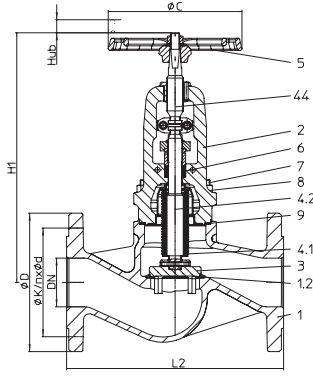
Fig. 141....154 1 1/2" - 6 zweiteilige Spindel
