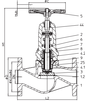
Fig. 141....112 1 1/2" - 6" zweiteilige Spindel
