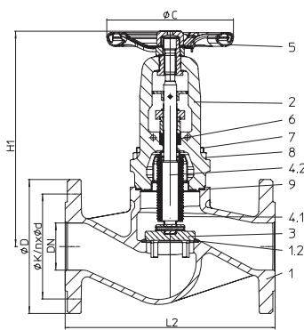
Fig. 141....153 1 1/2" - 6 einteilige Spindel
